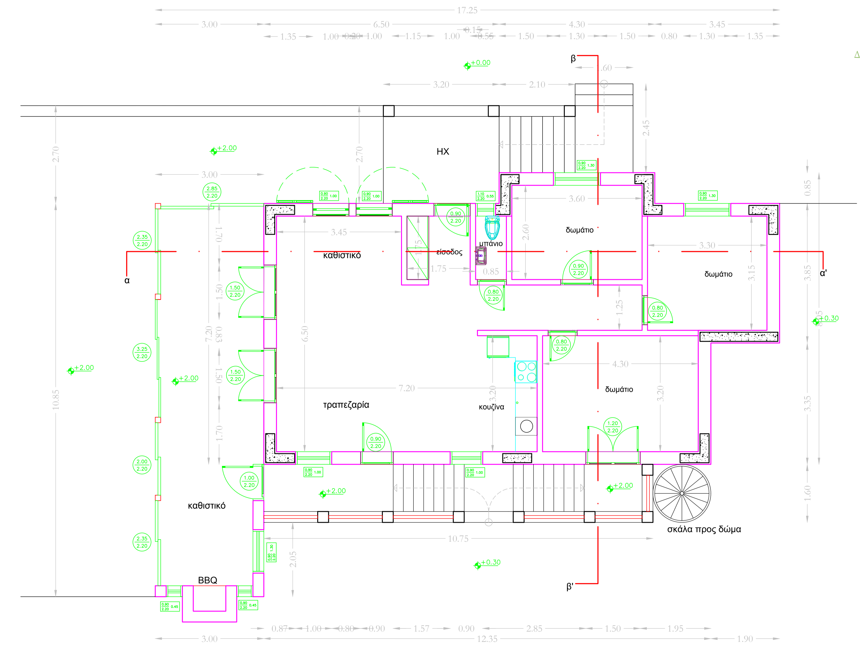
κάτοψη 2ης στάθμης
