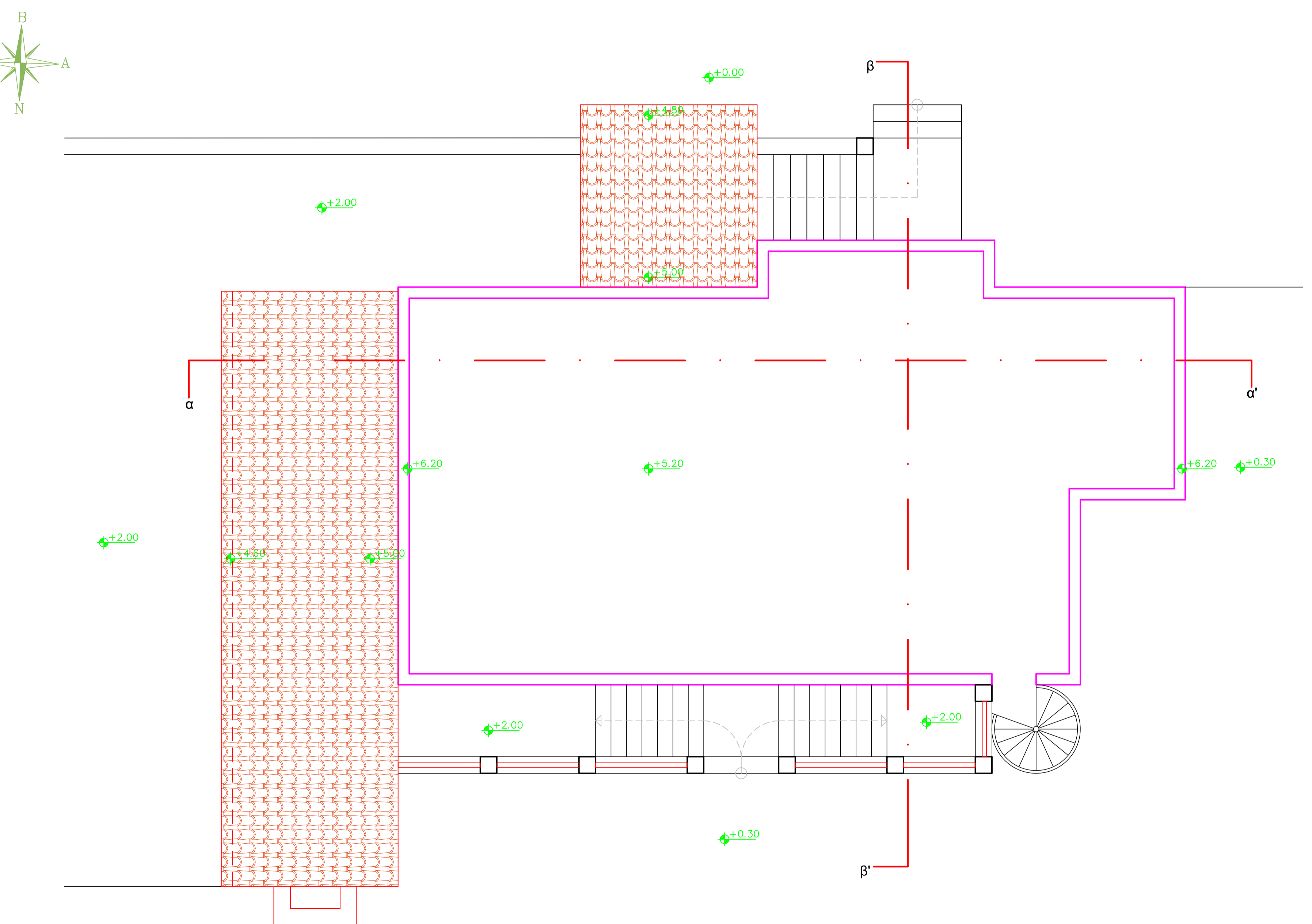
κάτοψη δώματος-στεγής
