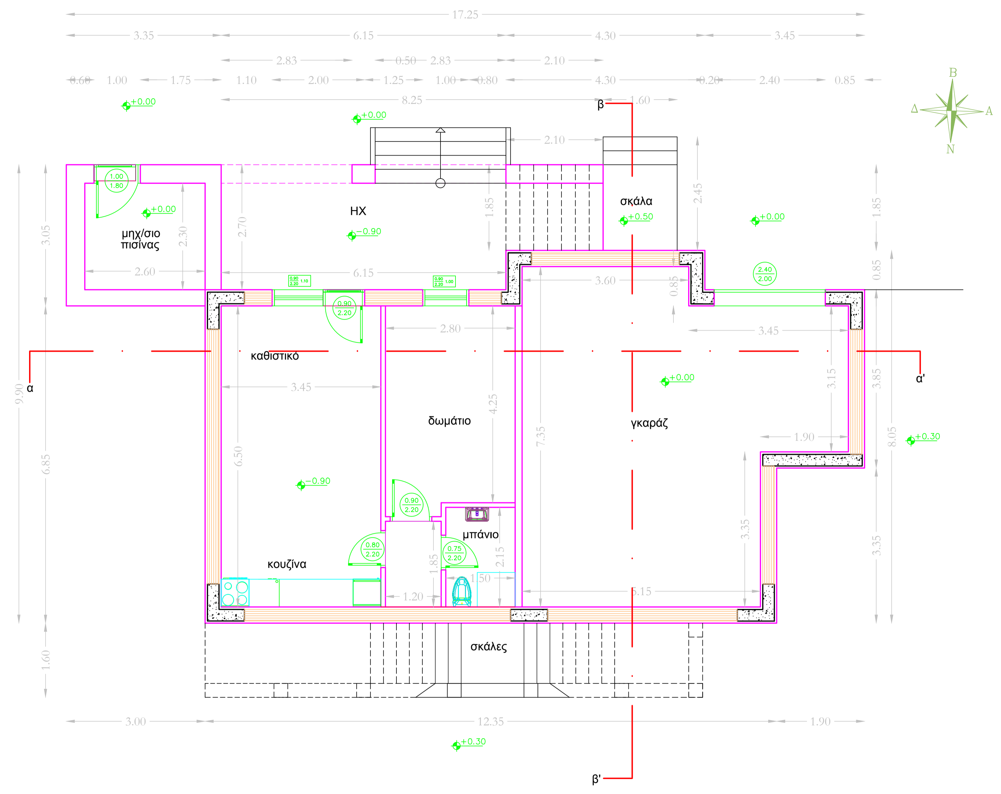
κάτοψη 1ης στάθμης
