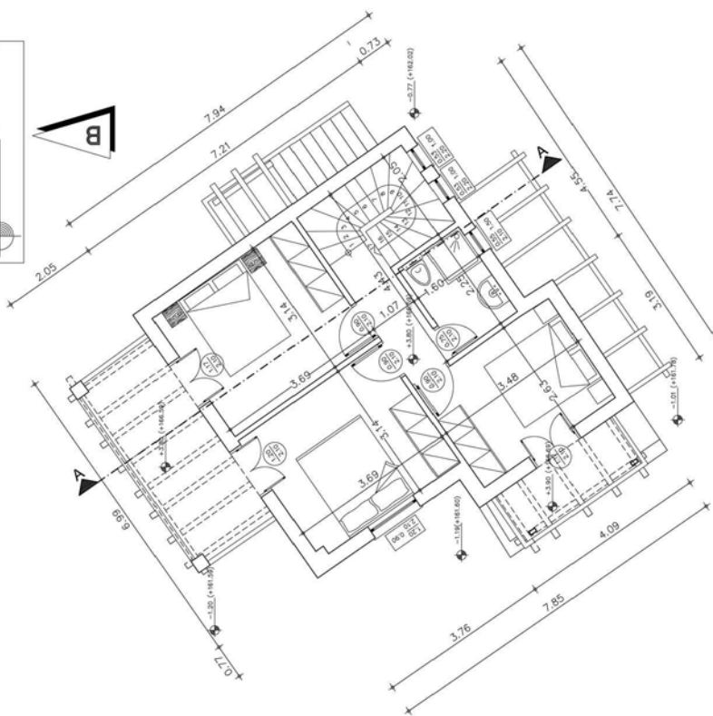
ΚΑΤΟΨΗ ΟΡΟΦΟΥ
