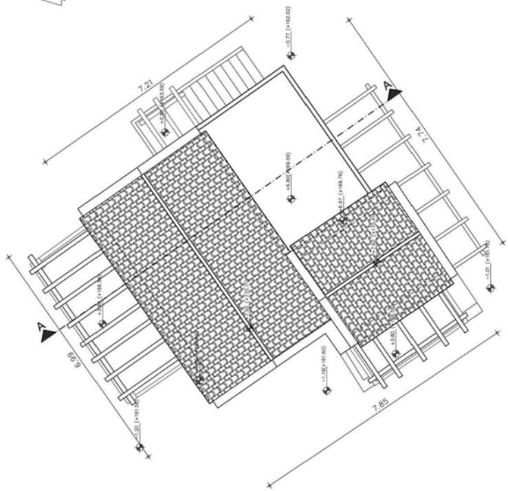
ΚΑΤΟΨΗ ΔΩΜΑΤΟΣ
