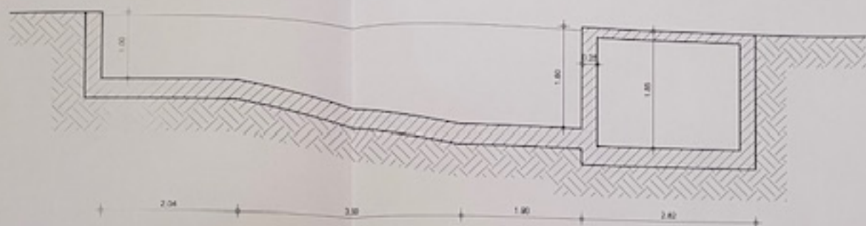
ΤΟΜΗ ΚΟΛΥΜΒΗΤΙΚΗΣ ΔΕΞΑΜΕΝΗΣ
